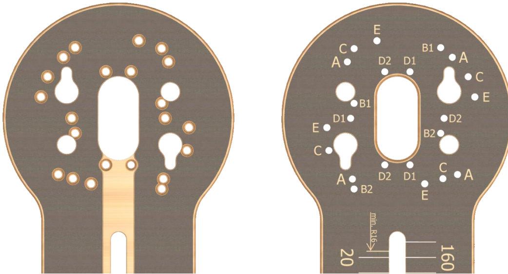
6Figura - Orificios de montaje para el módulo de router GKF600 de Bosch (imágenes a continuación)
