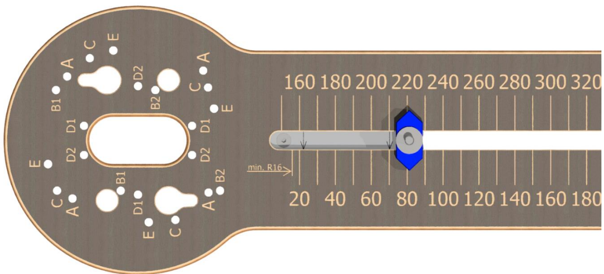
1Figura - Las flechas del carro deslizante apuntan a la escala inferior
