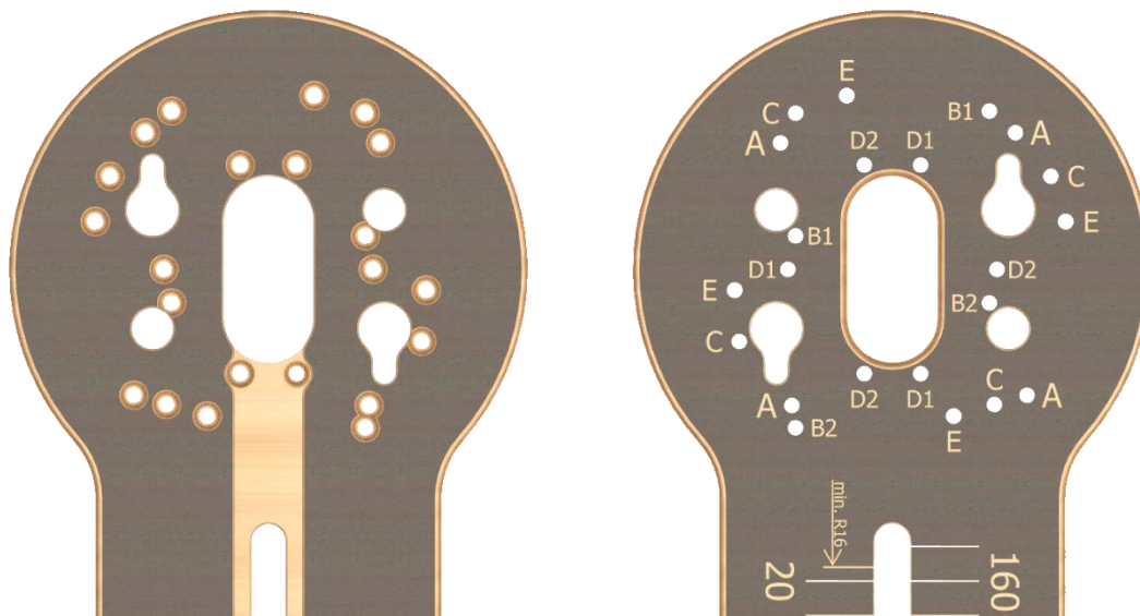
Figura 8- Orificios de montaje para el módulo de fresado angular B2 GKF600 de Bosch (imágenes siguientes)
