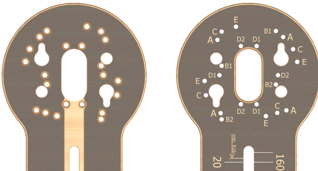
Figura 7- Orificios de montaje para el módulo de fresado acodado B1 GKF600 de Bosch (imágenes siguientes)
