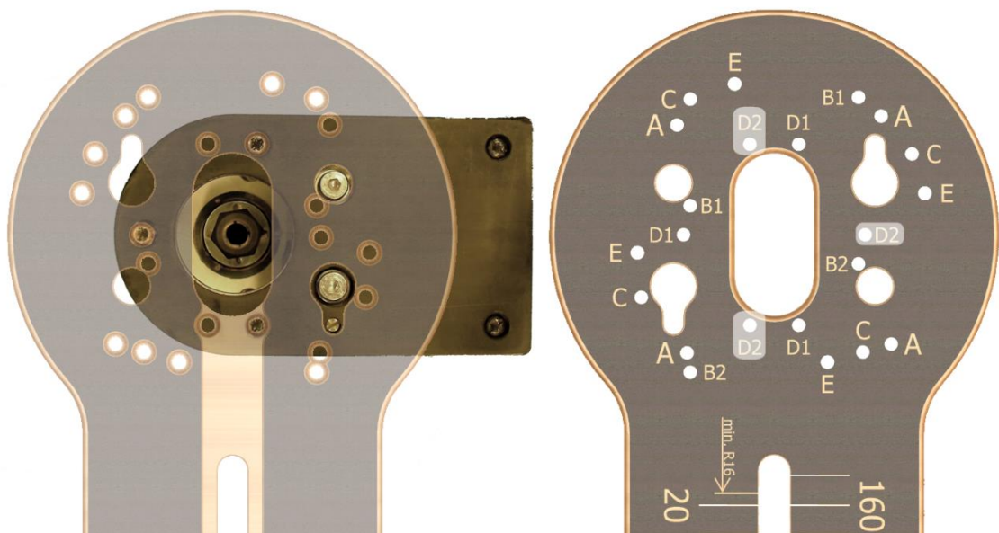
Figura 11- Montaje del GKF12V para diestros
