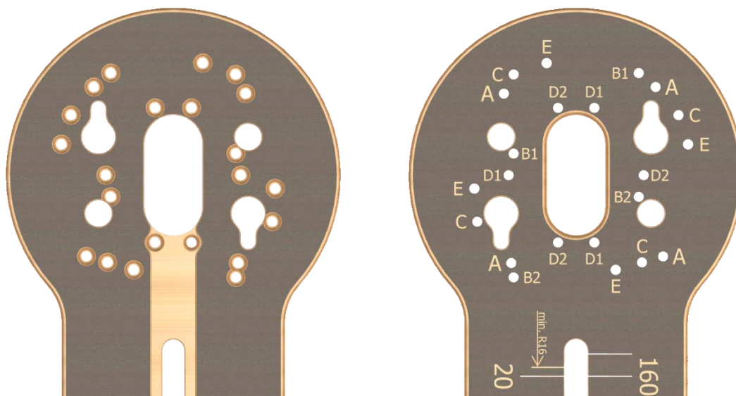
Figure 8- Trous de montage pour le module de fraisage angulaire B2 Bosch GKF600 (images à suivre)
