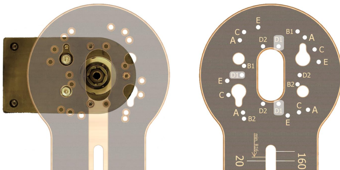
Figure 10- Montage GKF12V pour gauchers
