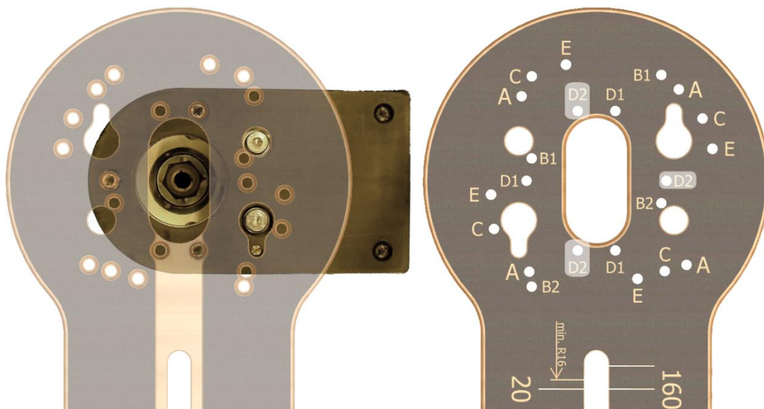
Figure 11- Montage du GKF12V pour droitiers
