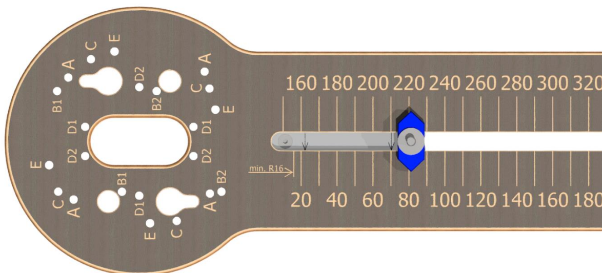
Figure1 - Les flèches de la glissière pointent vers l'échelle inférieure
