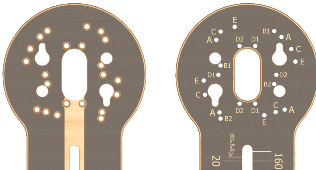
Figure 9- Trous de montage pour le module de fraisage de chants C Bosch GKF600 (images à suivre)
