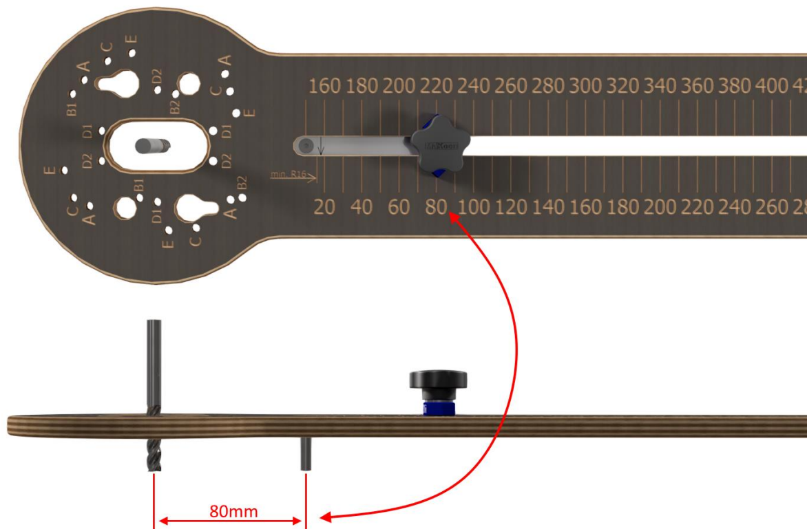
Illustration3 - Illustration d'une mesure réglée, ici 80mm
