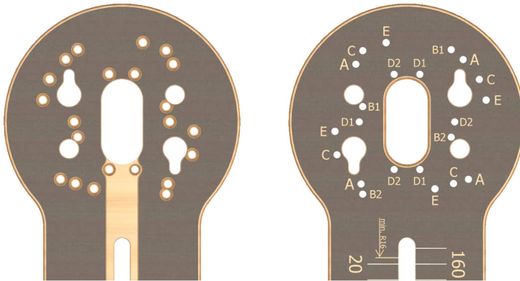
Illustration6 - Trous de montage pour module de défonçage GKF600 Bosch (images à venir)
