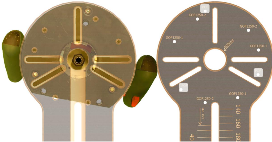
Figura 6- Orificios de montaje para el POF 1400 de Bosch
