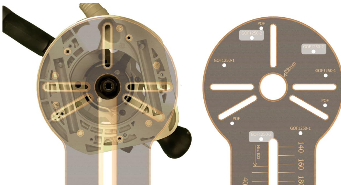
Figura 8- Orificios de montaje para Bosch GOF 1250-2
