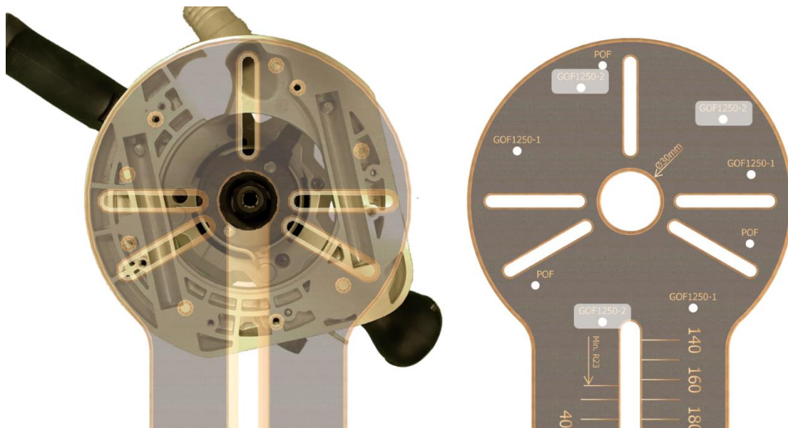
Figure 8- Trous de montage pour Bosch GOF 1250-2
