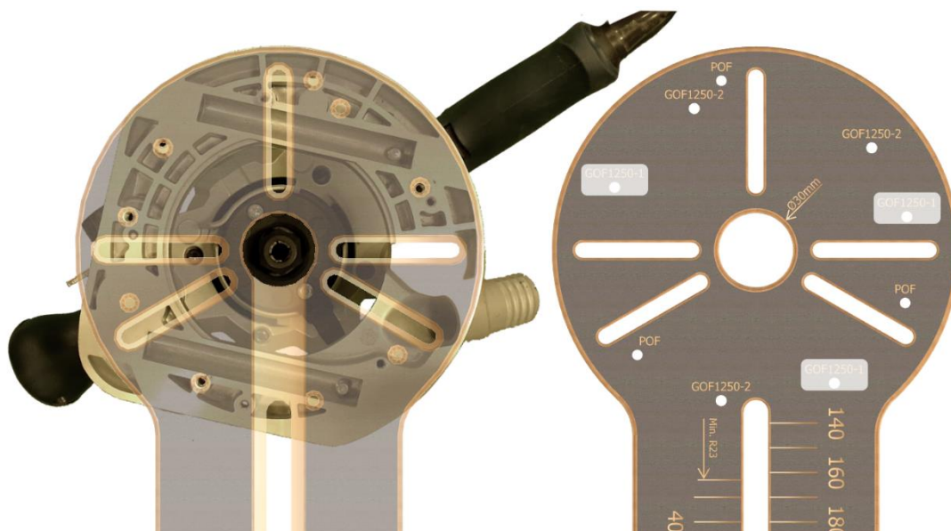
Figure 7- Trous de montage pour Bosch GOF 1250-1
