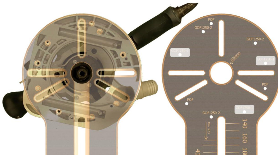
7attēls - Bosch GOF 1250-1 montāžas atveres
