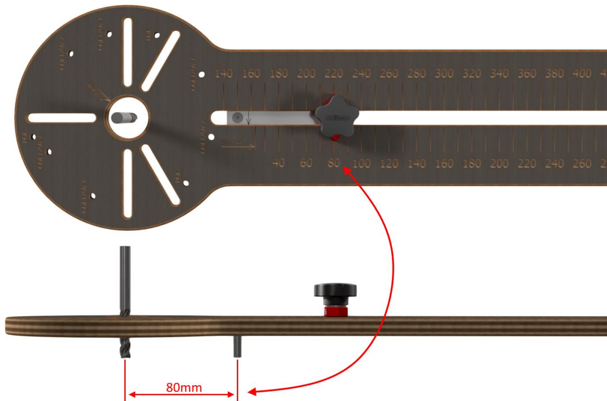
Figuur 3- Illustratie van een ingestelde afmeting, hier 80 mm
