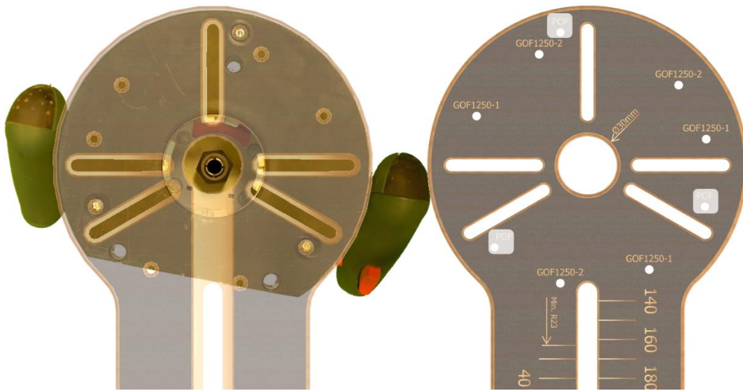
Afbeelding 6- Montagegaten voor Bosch POF 1400
