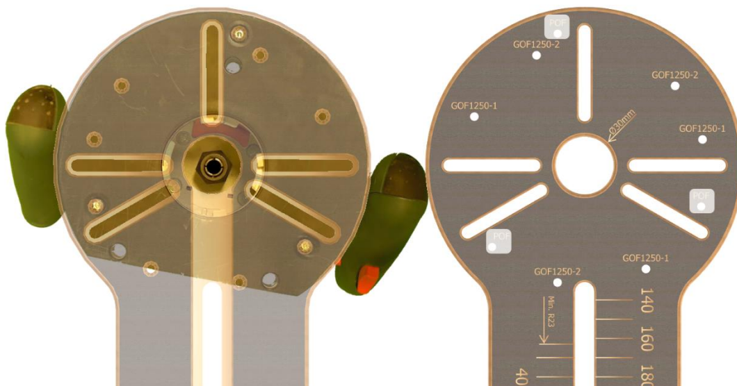
Obrázok 6- Montážne otvory pre Bosch POF 1400
