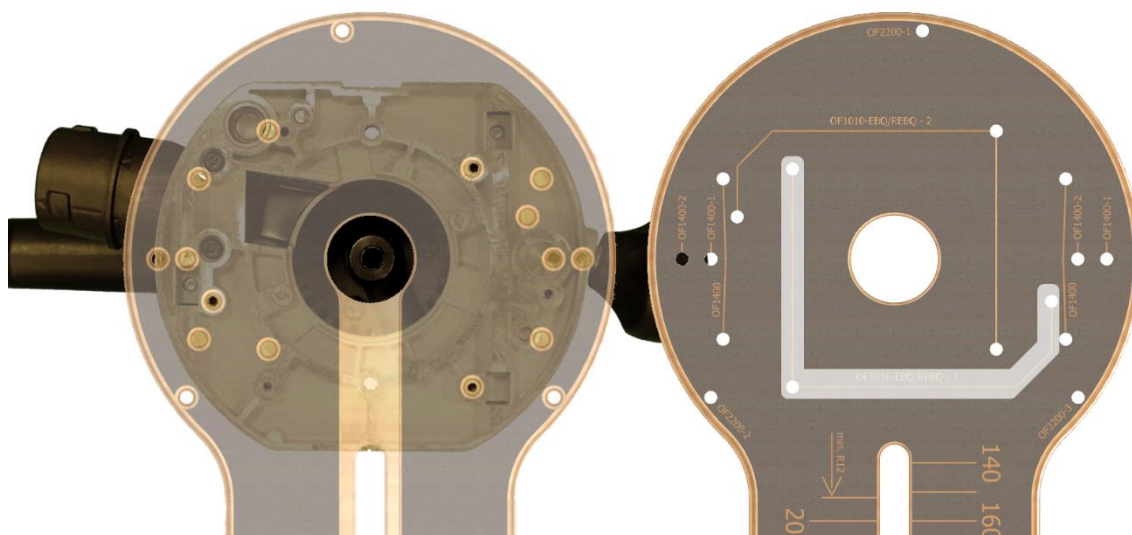
7Attēls - Stiprinājuma atveres 1, kas piemērotas Festool OF1010-REBQ
