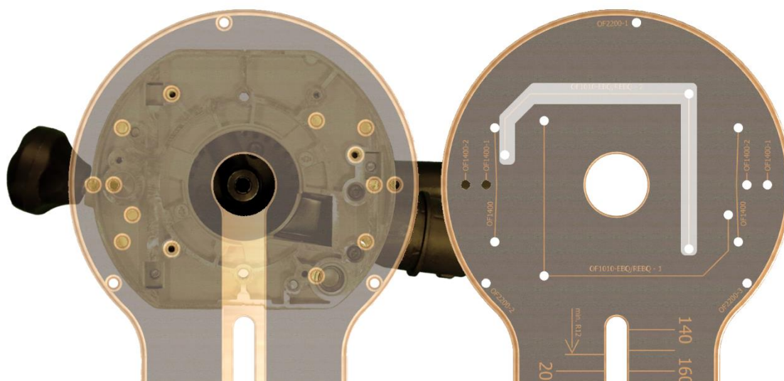
9attēls - Stiprinājuma atveres 2, kas piemērotas Festool OF1010-REBQ
