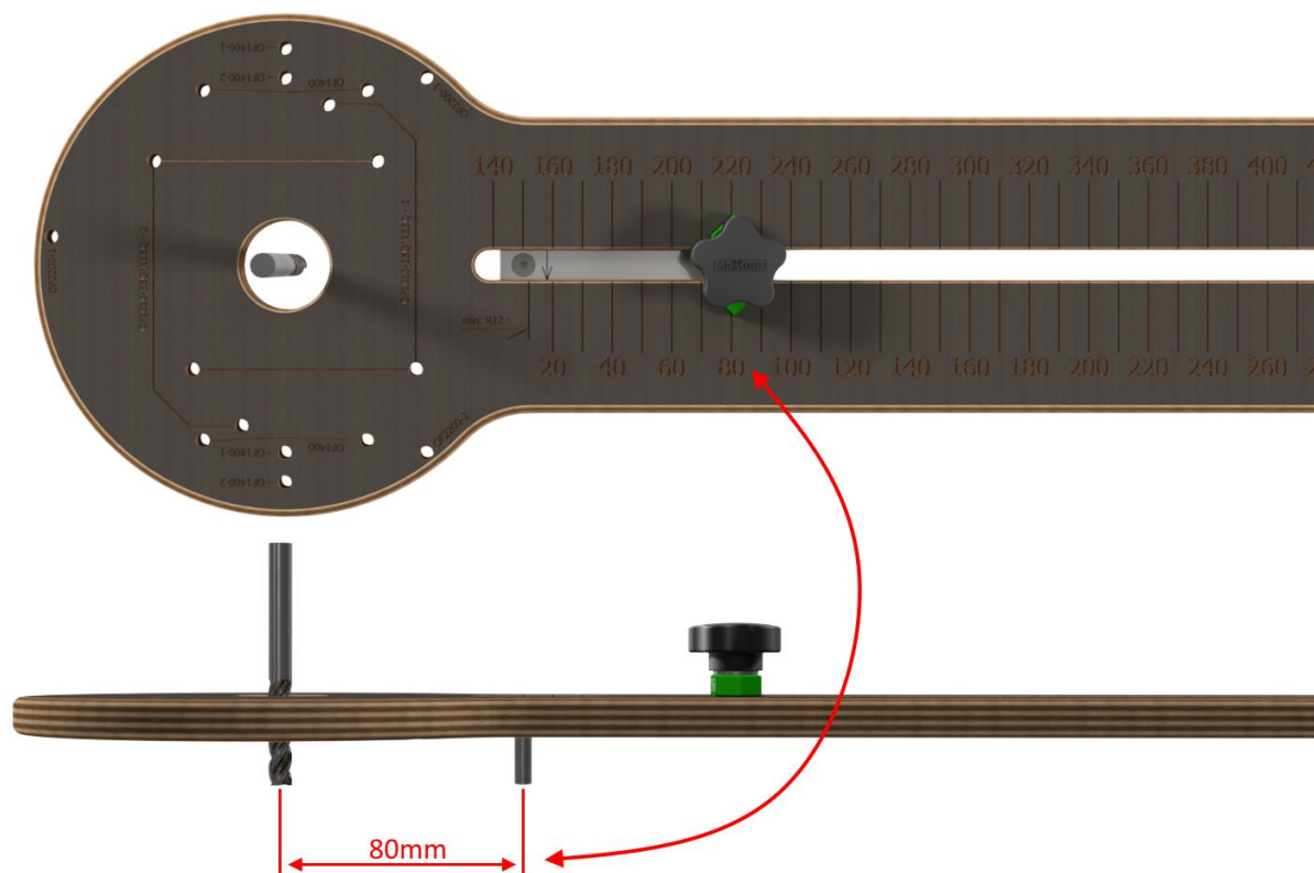
3attēls - Uztādītā izmēra ilustrācija, šajā gadījumā 80 mm.
