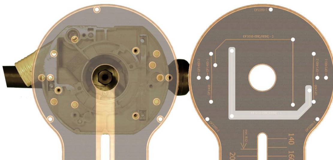
6Attēls - Stiprinājuma atveres 1, kas piemērotas Festool OF1010-REB
