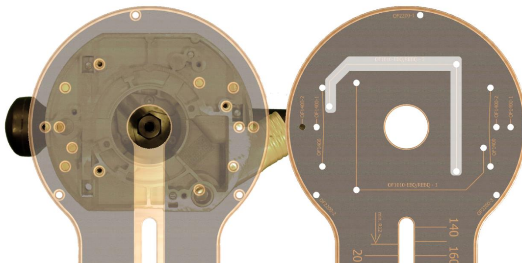
8attēls - Stiprinājuma atveres 2, kas piemērotas Festool OF1010-REB
